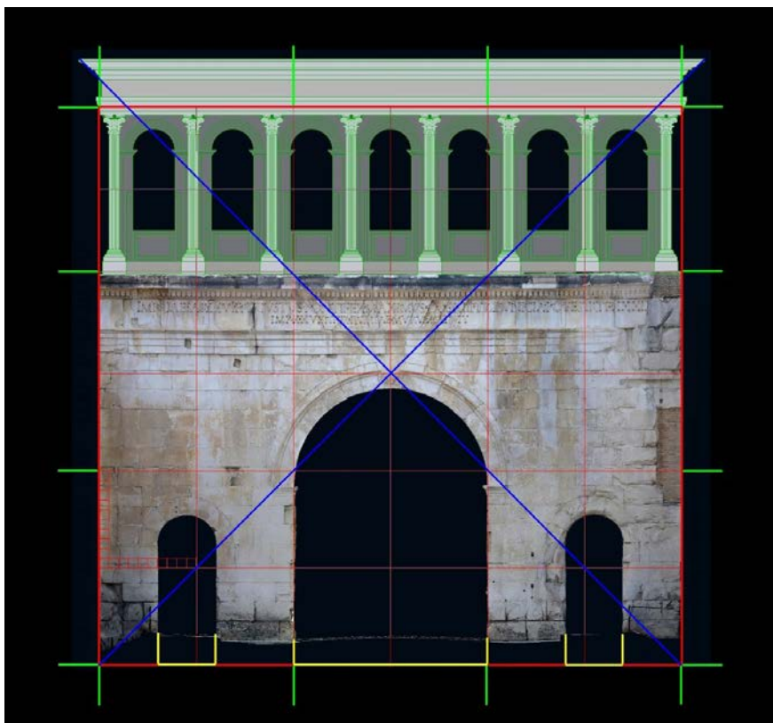
Figura 6. Porta di Augusto di Fanum Fortunae, rilievo fotogrammetrico e ricostruzione dell'attico con indicazione dei rapporti esistenti tra le membrature architettoniche (elaborazione: L. Baratin e G. Checcucci).
