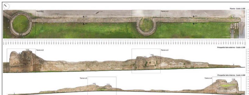
Fig. 6 – Tavole tecniche CAD.
