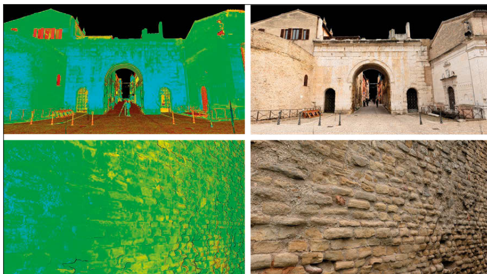
Fig. 4 – Campionamento ad alta densità ottenuto da laser scanner.
